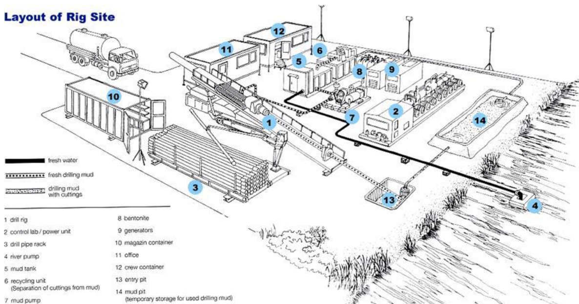
Фигура 6 Принципна схема на разполагане на монтажното оборудване на сондажната площадка
