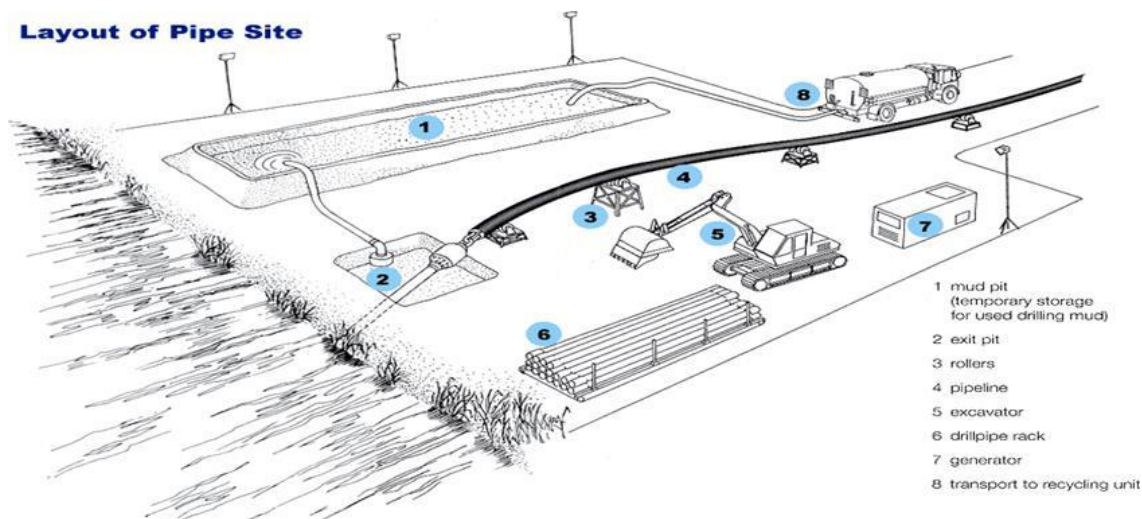
Фигура 7 Принципна схема на тръбната площадка за направа на дюкер
